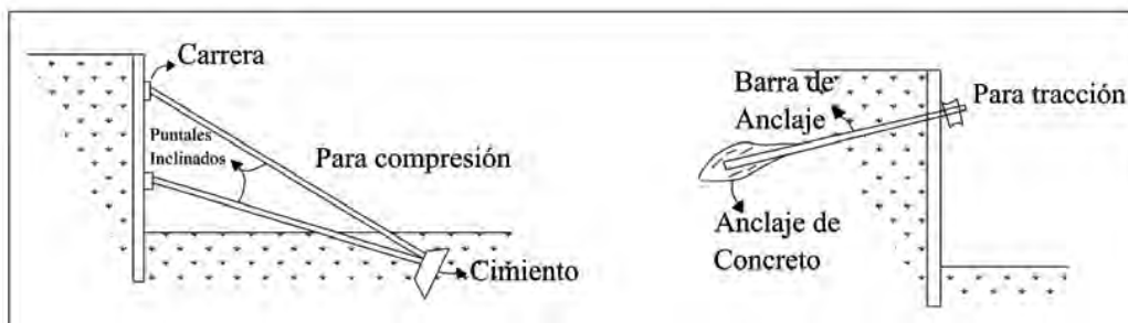
Puntales inclinados con Cimentación temporal
